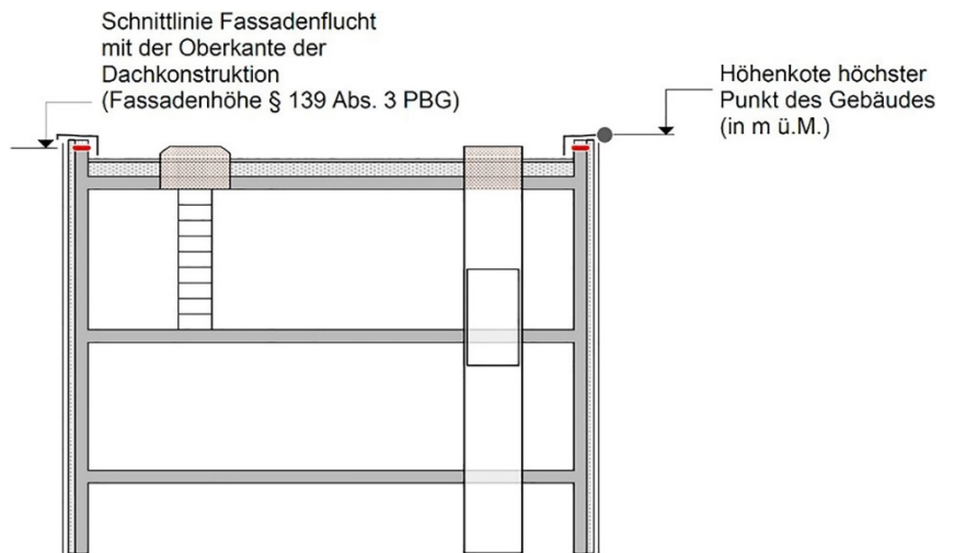
Abbildung 52: Skizze zum massgebenden höchsten Punkt der Dachkonstruktion bei Flachdächern
