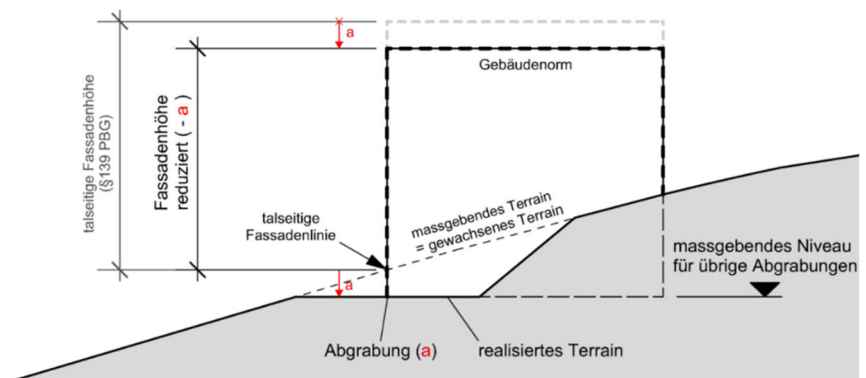
Abbildung 55: Skizze Reduktion der talseitigen Fassadenhöhe bei Abgrabungen am Gebäude
