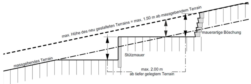
Abbildung 47: Skizze Terraingestaltung (Art. 9 BZR)
