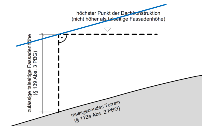
Abbildung 53: Skizze zur talseitigen Fassadenhöhe und Regelung zum höchsten Punkt der Dachkonstruktion, der nicht höher als die talseitige Fassadenhöhe liegen darf (parallel zum massgebenden Terrain).
