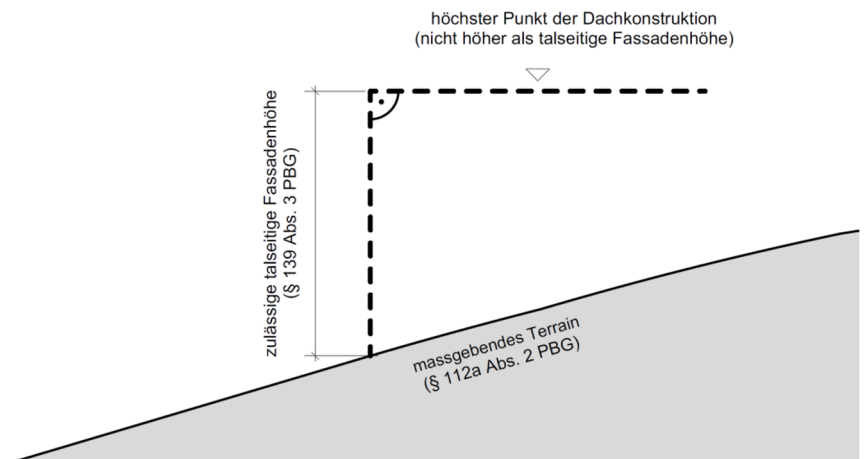
Abbildung 50: Skizze zur talseitigen Fassadenhöhe und Regelung zum höchsten Punkt der Dachkonstruktion, der nicht höher als die talseitige Fassadenhöhe liegen darf.
