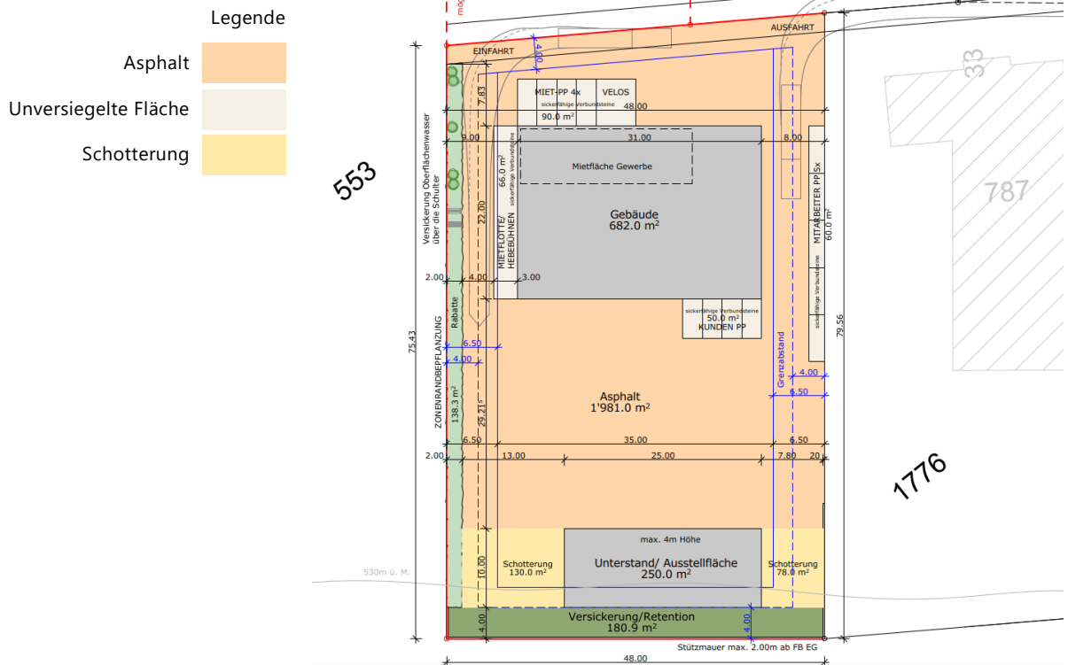
Abbildung 19: Flächenverteilung auf dem geplanten Betriebsareal. | Quelle: massplan AG
