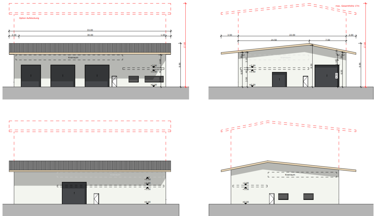
Abbildung 9: Aussenansicht des geplanten zweigeschossigen Gewerbebaus. | Quelle: massplan AG
