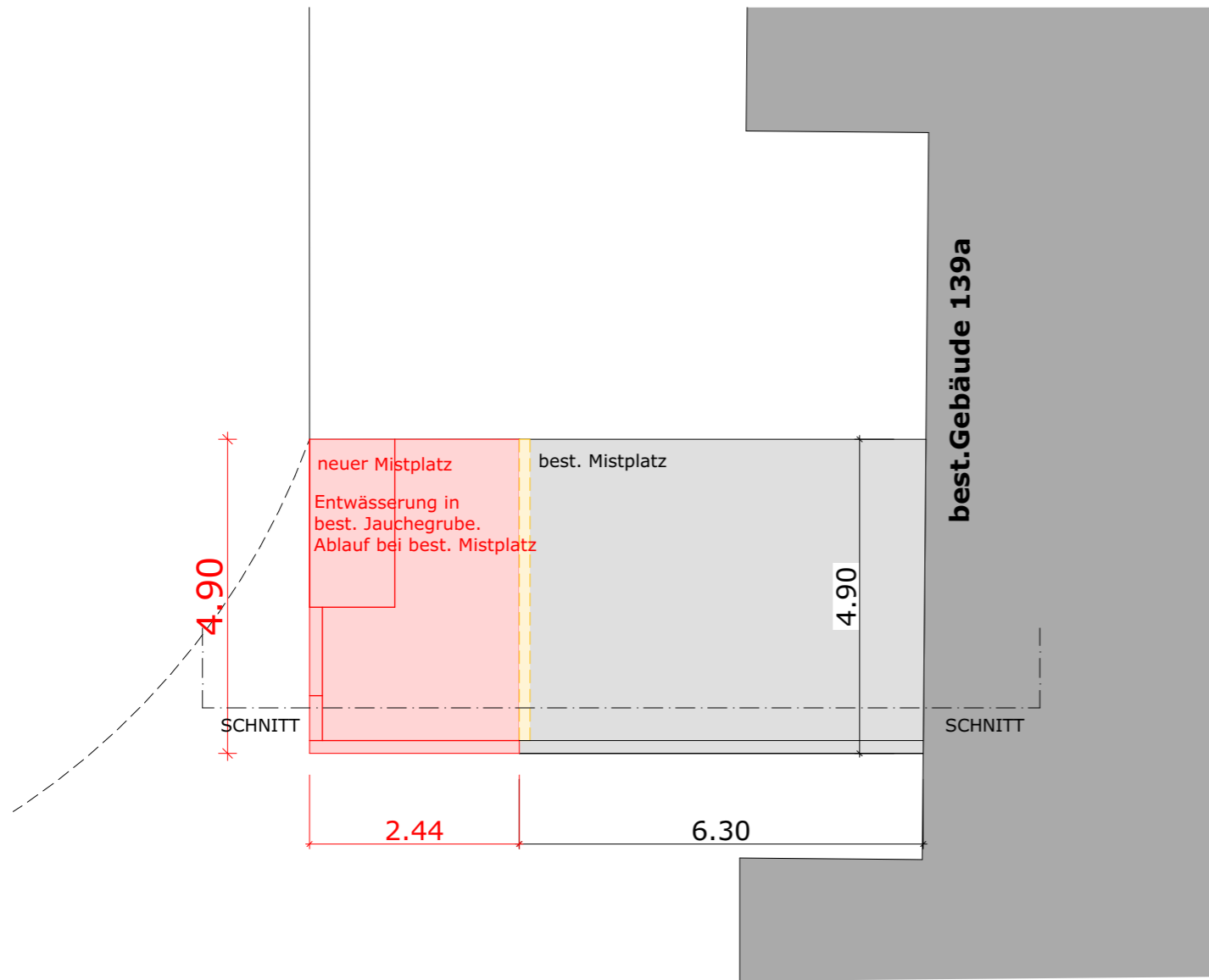
GRUNDRISS
